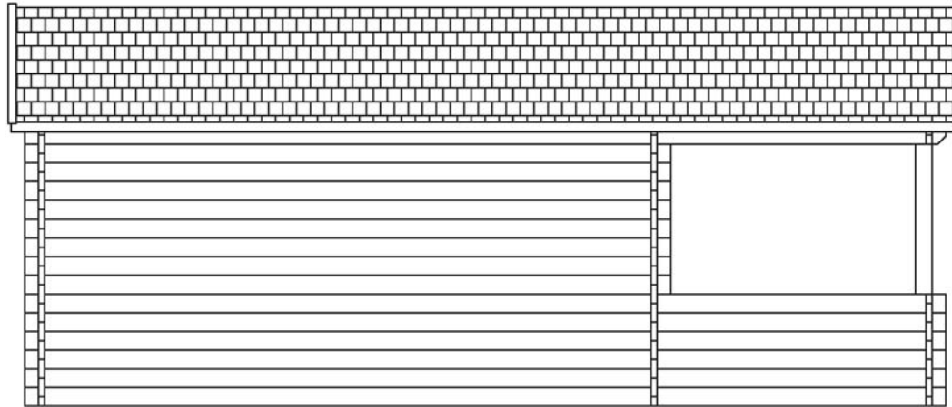
Ansicht links / left view
